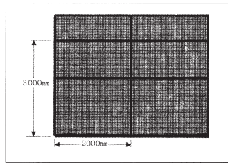
落石防護柵
