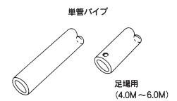
単管パイプ 足場用 (4.0M~6.0M) ピン無し 仮設用 (バタ用) (0.5M~6.0M) φ48.6×2.4炭素鋼管
